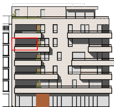
VOORGEVEL NIEUWPOORTSESTEENWEG
